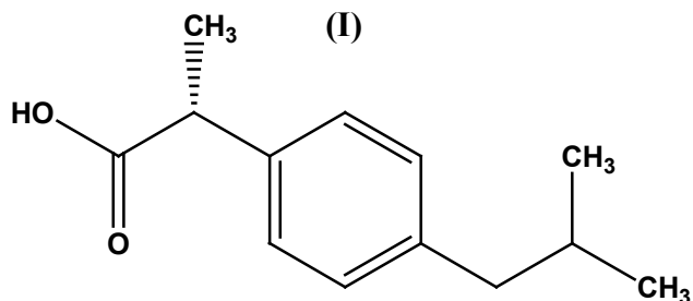
(R)-Ibuprofeno
