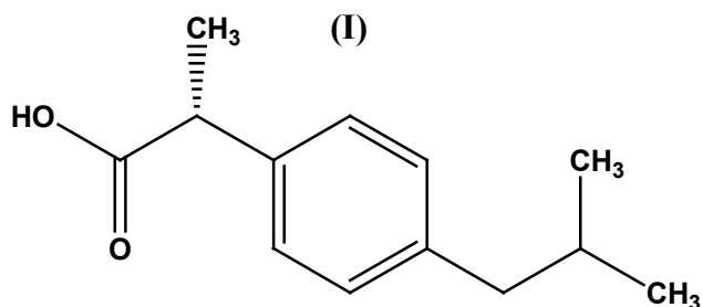
(R)-Ibuprofeno
